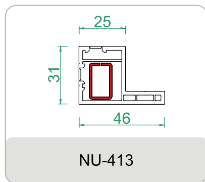
GRILL FRAME
